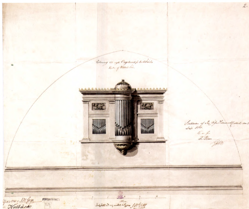
Fig. 2. Ritning till Orgelverk i Kolbäcks kyrka av arkitekt Jacob Wilhelm Gerss (1784–1844), godkänd av Överintendents-ämbetet 3 maj 1840. Originalen i Riksarkivet. Foto Tomas Svenske.
