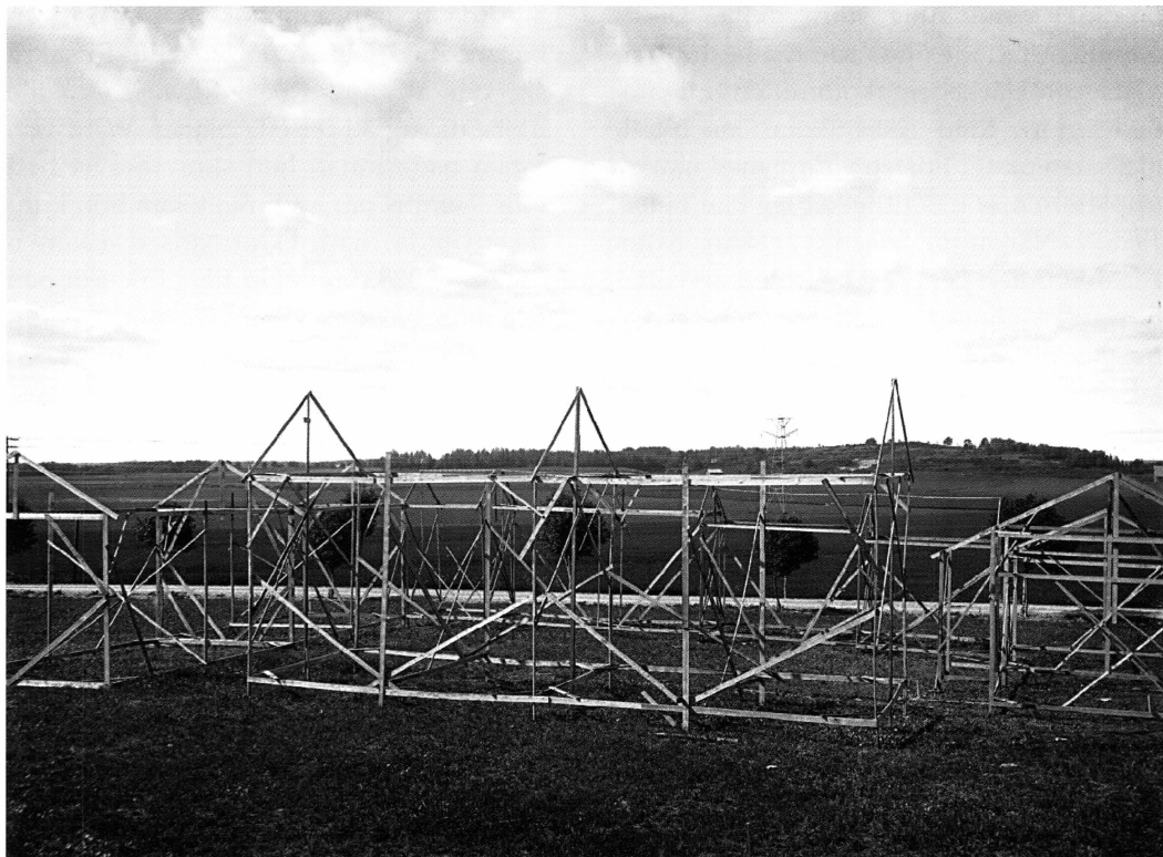
Brädmodeller av de olika husen sattes upp under sommaren 1928. På så sätt kunde man få en bra utvärdering av olika sätt att disponera området. Foto Paul Sandberg. PS06823.
