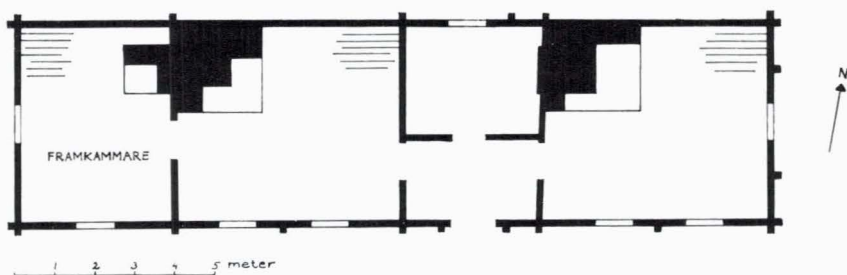
Bild 1. Plan av framkammарstuga vid Byle gård, Funbo socken. Rekonstruktion av Ulrich Lange efter uppmättningsritning och fotografier av Carl Lennart Ceder. Byggnaden uppfördes i ett sammanhang omkr. 1790. Lägga märke till den nästan fönsterlösa norra väggen.
