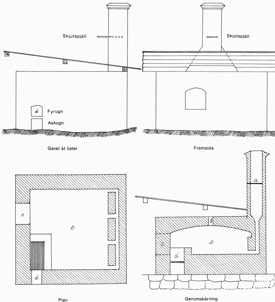
Bild 3. Tempelugn vid Sigtuna Glasbruk. Renritning av original i Sigtuna rådstuvurätts dombok 1885.
