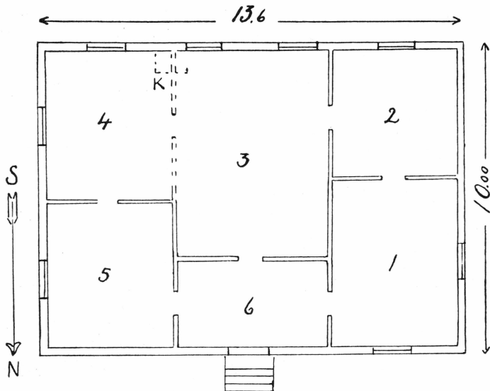
Bild 2. Sockenskolans bottenplan. 1. Lärarens kök; 2, 4 och 5. Lärarens rum; 3. Skolsal; 6. Förstuga. (Fr. o. m. 1852 användes 3 och 4 som skolsal; väggen togs bort, kateder vid K.)
