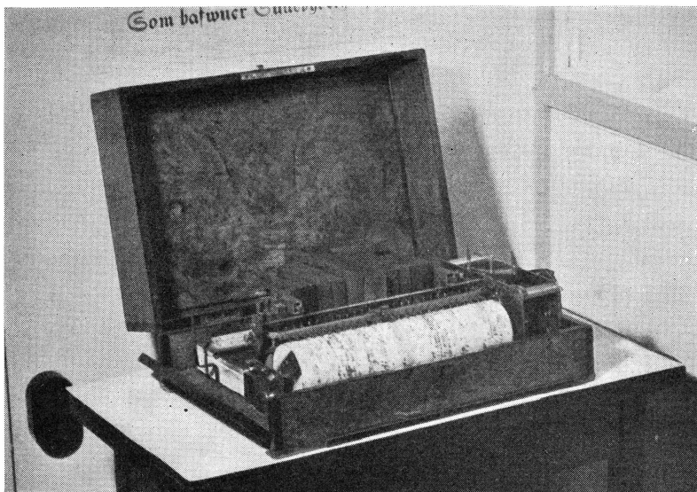
Bild 1. Serinett från 1800-talets början.
